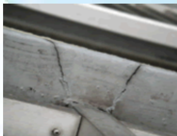
鼻先天端ひび割れ
