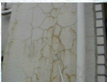
亀甲状のひび割れと浮き
